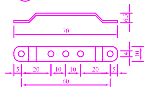
① 一자 브라켓
